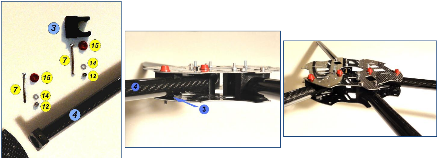
Éléments de montage/Assembly parts
