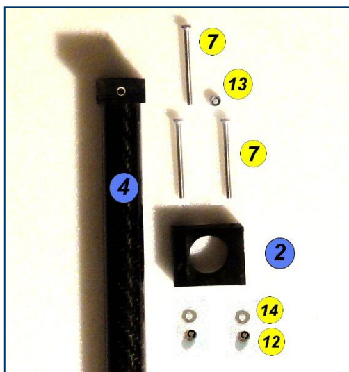
Éléments de montage/Assembly parts
